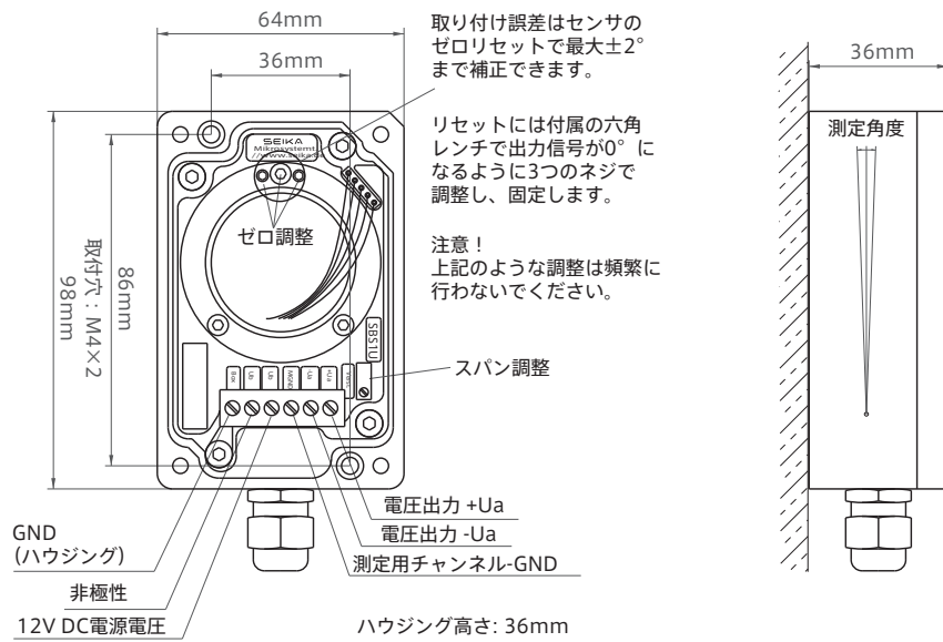
外形寸法図
