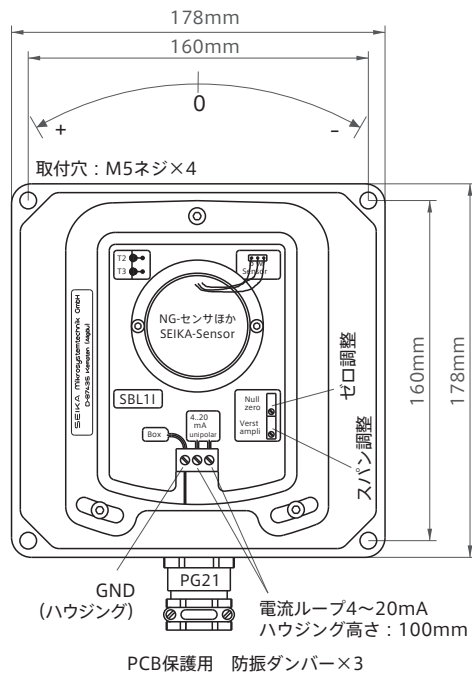
外形寸法図
