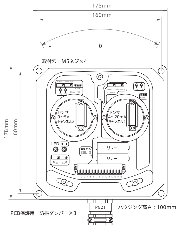
外形寸法図
