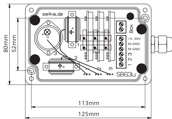
外形寸法図
