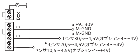
接続図
