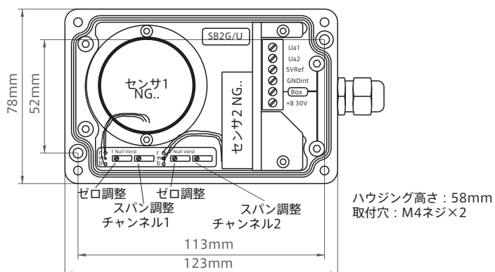
外形寸法図
