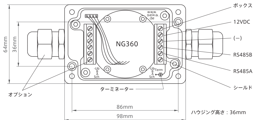
外形寸法図
