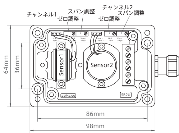
外形寸法図
