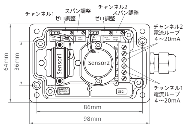
外形寸法図
