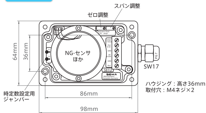
外形寸法図
