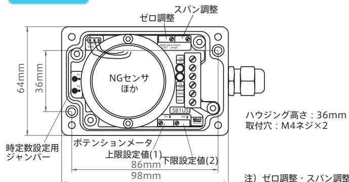
外形寸法図
