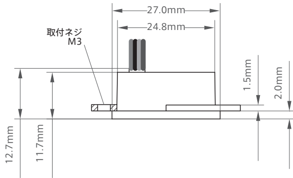
外形寸法図
