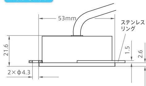
外形寸法図
